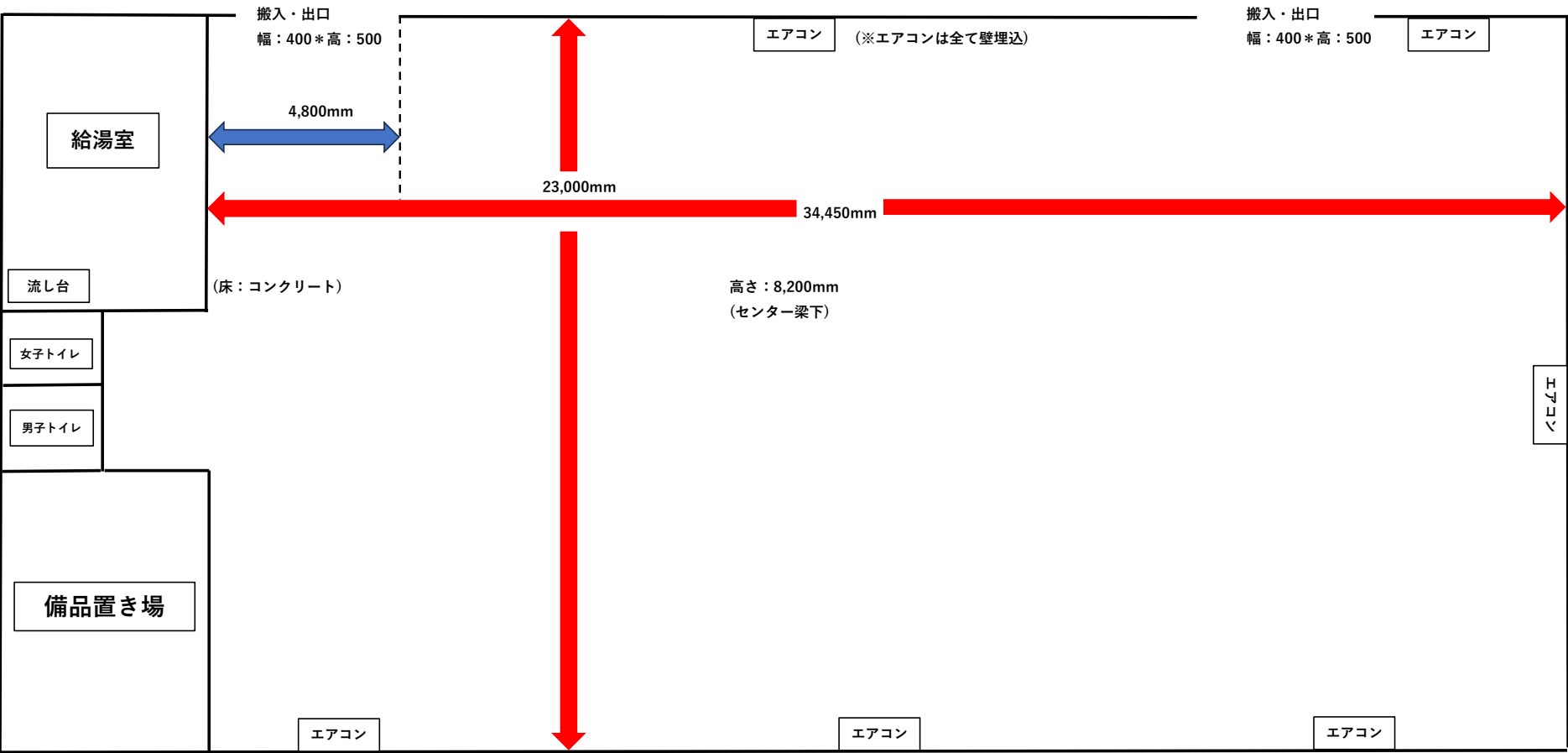
【下戸田創庫稽古場図面】
