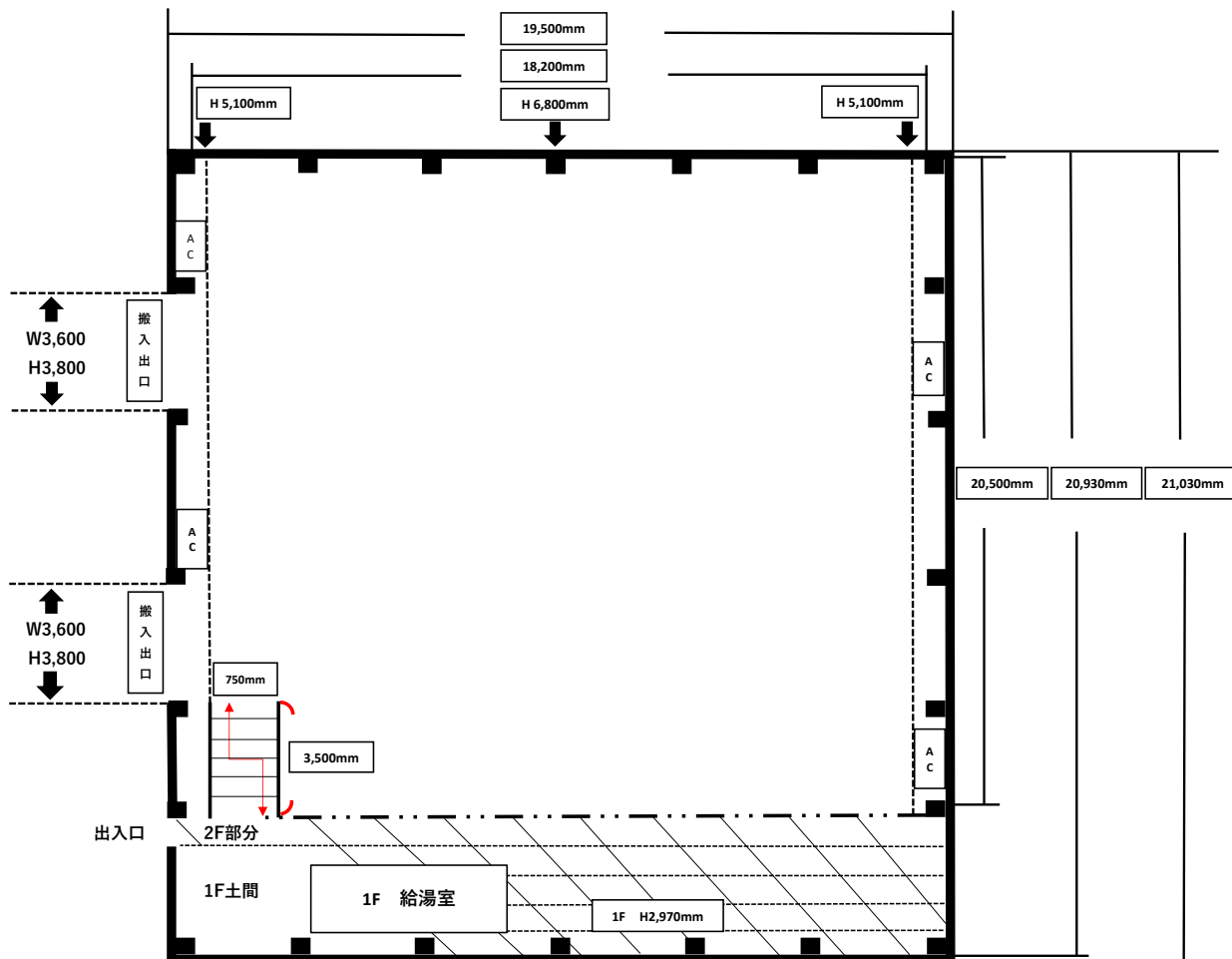
【第5創庫稽古場図面】
